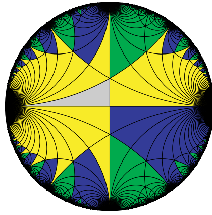
(b) W_{23\infty}
